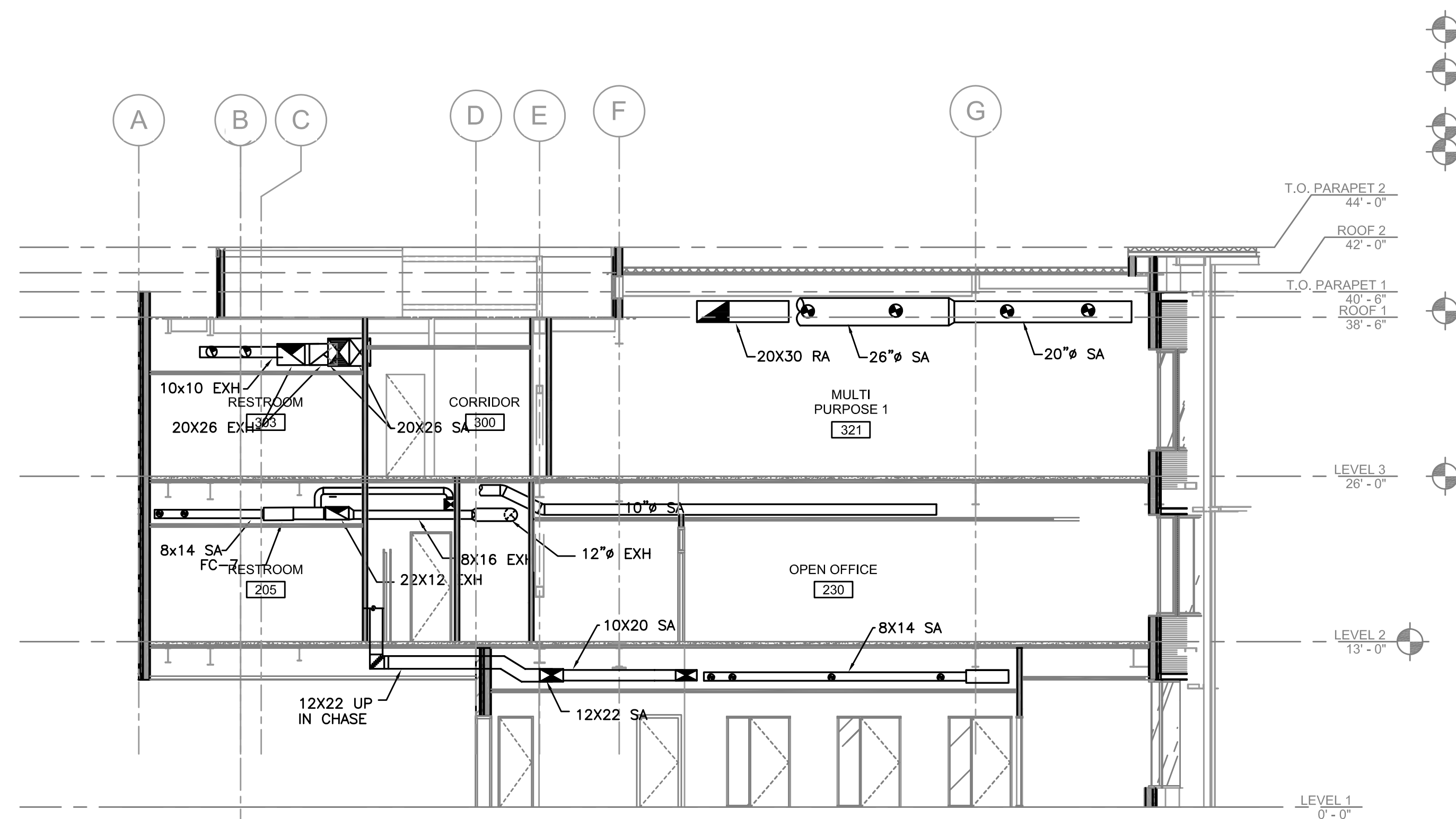
1 HVAC SECTION 'B' M4.01 SCALE:
